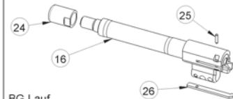
BG Lauf
