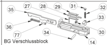
BG Verschlussblock
