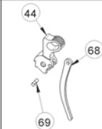
BG Schlaghahn
